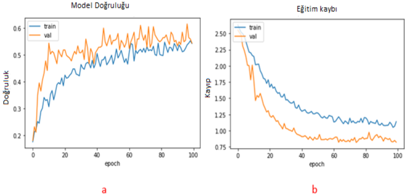
Şekil 4. Nokta Bulutu modeli performans grafikleri a) model doğruluğu grafiği b) eğitim kayıp grafiği
